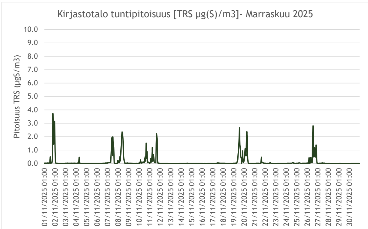
Kuva 4. TRS-tuntipitoisuudet ( \mu\text{gS}/\text{m}^3 ) Kirjastotalolla -Marraskuu 2025.
