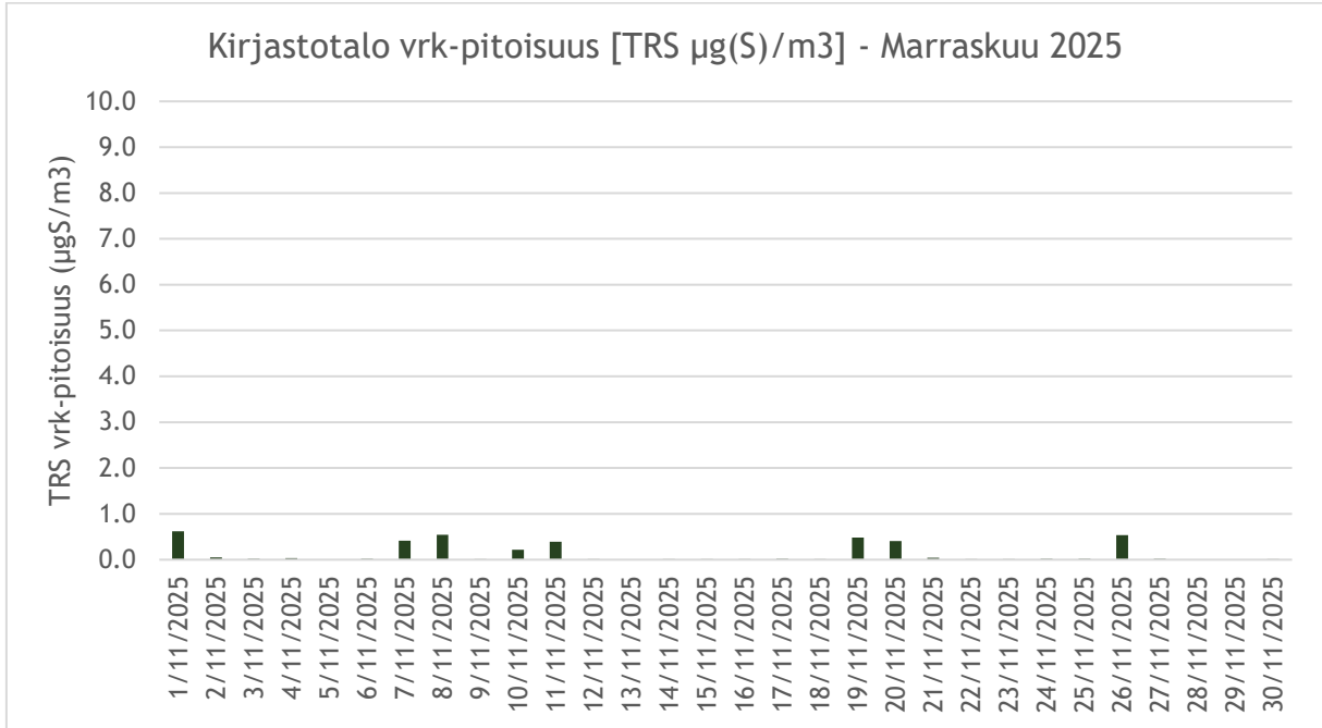
Kuva 3. TRS-vuorokausipitoisuudet ( \mu\text{gS}/\text{m}^3 ) -Marraskuu 2025. Vuorokausiohjearvo on 10 \mu\text{gS}/\text{m}^3
