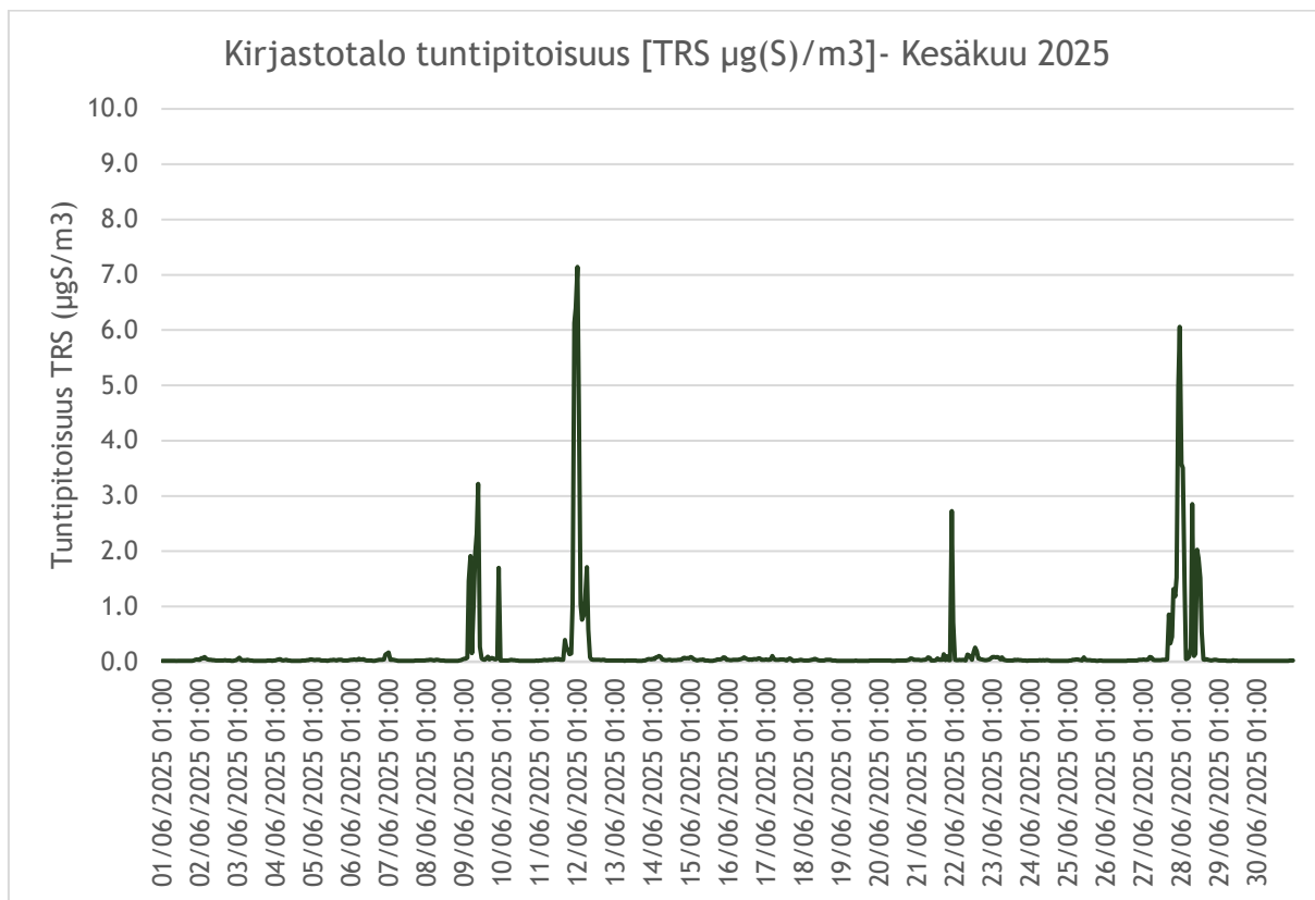
Kuva 4. TRS-tuntipitoisuudet ( \mu\text{gS}/\text{m}^3 ) Kirjastotalolla -Kesäkuu 2025.
