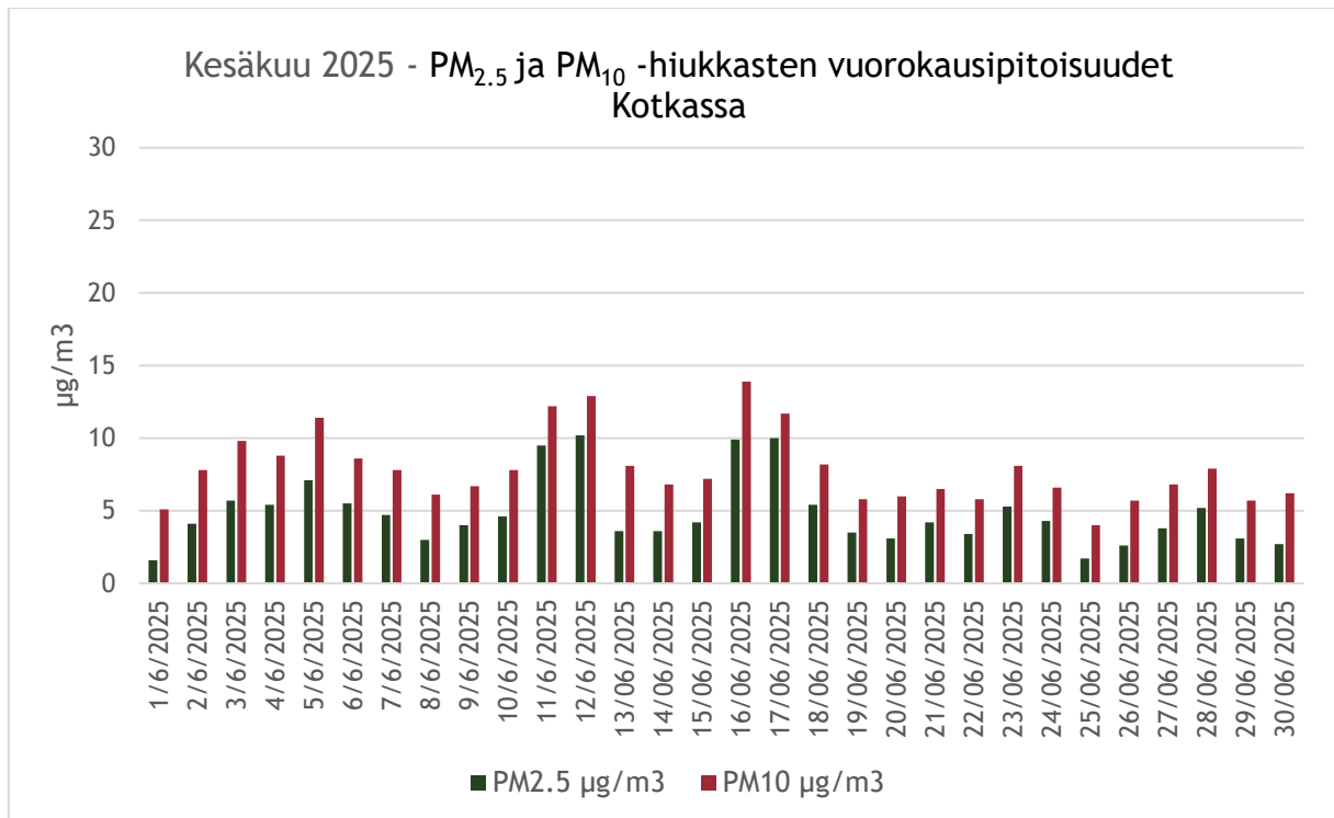
Kuva 2. Kirjastotalon PM 2.5 ja PM 10 -hiukkasten vuorokausipitoisuudet (µg/m 3 ) - Kesäkuu 2025. PM 10 kansallinen vrk-ohjearvo on 70 µg/m 3 ja vrk:n raja-arvon lukuarvo 50 µg/m 3 . WHO:n PM 10 vrk-ohjearvo on 45 µg/m 3 , PM 2.5 vuosiohjearvo on 5 µg/m 3 ja vrk-ohjearvo 15 µg/m 3 . Uudistettu ilmanlaatuasetus voimaan 1.1.2030: PM 2.5 vrk-raja-arvo on 25 µg/m 3 ja PM 10 vrk-raja-arvo 45 µg/m 3
