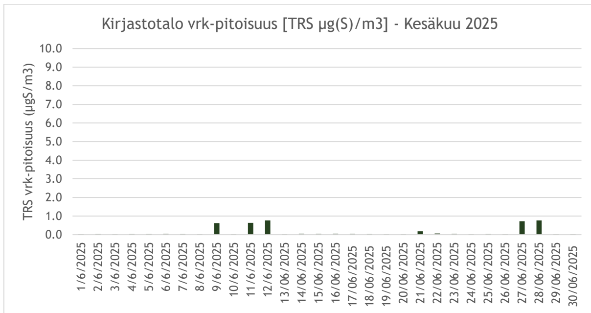
Kuva 3. TRS-vuorokausipitoisuudet ( \mu\text{gS}/\text{m}^3 ) -Kesäkuu 2025. Vuorokausiohjearvo on 10 \mu\text{gS}/\text{m}^3
