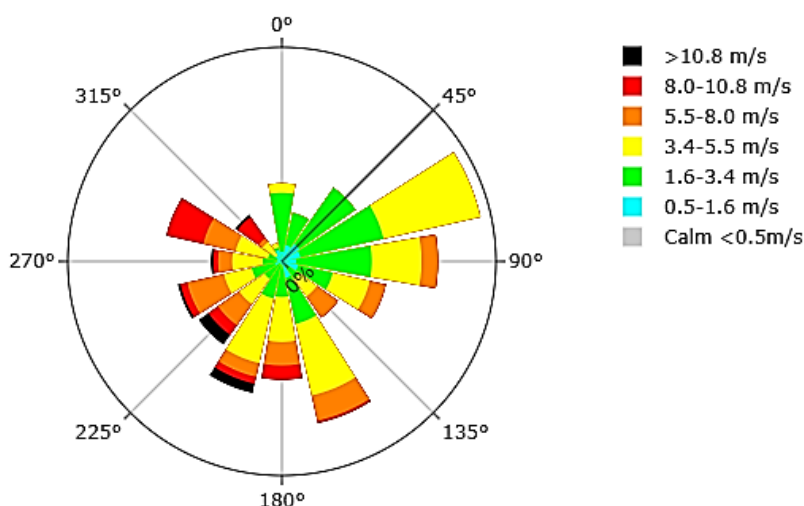
Kuva 1. Tuulen suunta- ja nopeusjakauma Kotkassa helmikuussa 2024. Tyyntä alle 0.5 m/s oli 0.1 % ajasta (Tuuliruuus = mistä tuulee).
