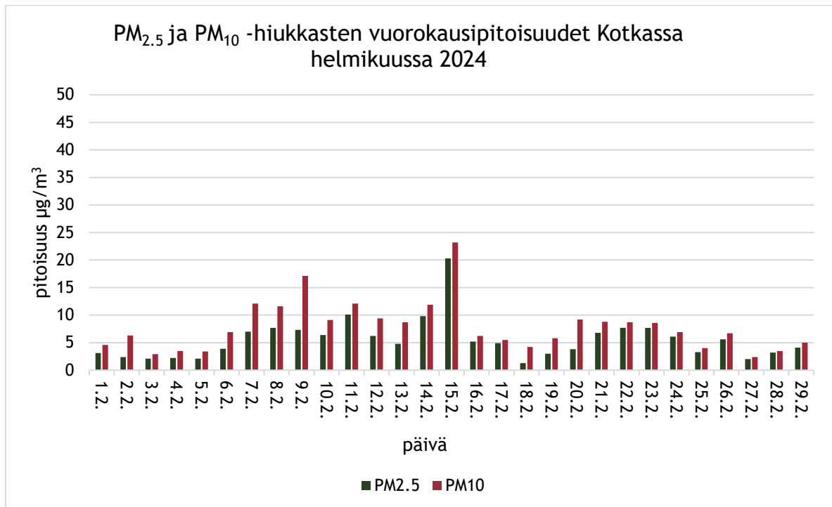
Kuva 2. Kirjastotalon PM 2.5 ja PM 10 -hiukkasten vuorokausipitoisuudet (µg/m 3 ) helmikuussa 2024. PM 10 vrk-ohjearvo on 70 µg/m 3 ja raja-arvon lukuarvo 50 µg/m 3 . WHO:n PM 10 vrk-ohjearvo on 45 µg/m 3 , PM 2.5 vuosiohjearvo on 5 µg/m 3 ja vrk-ohjearvo 15 µg/m 3 .
