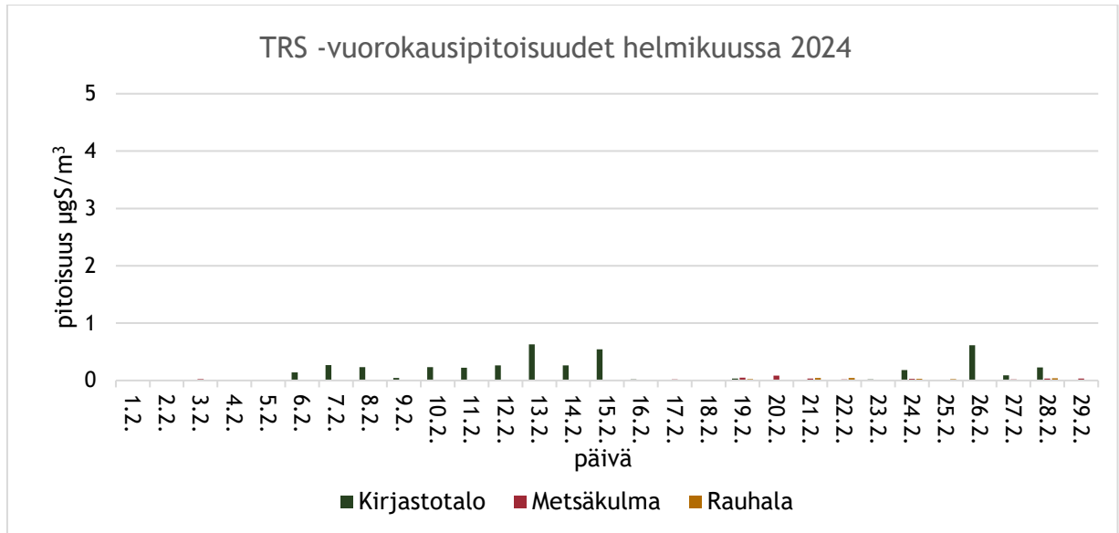
Kuva 3. TRS-vuorokausipitoisuudet ( \mu\text{gS}/\text{m}^3 ) helmikuussa 2024. Vuorokausiohjearvo on 10 \mu\text{gS}/\text{m}^3 (vertailuarvo kk:n 2. korkein = 0.2 \mu\text{gS}/\text{m}^3 ).
