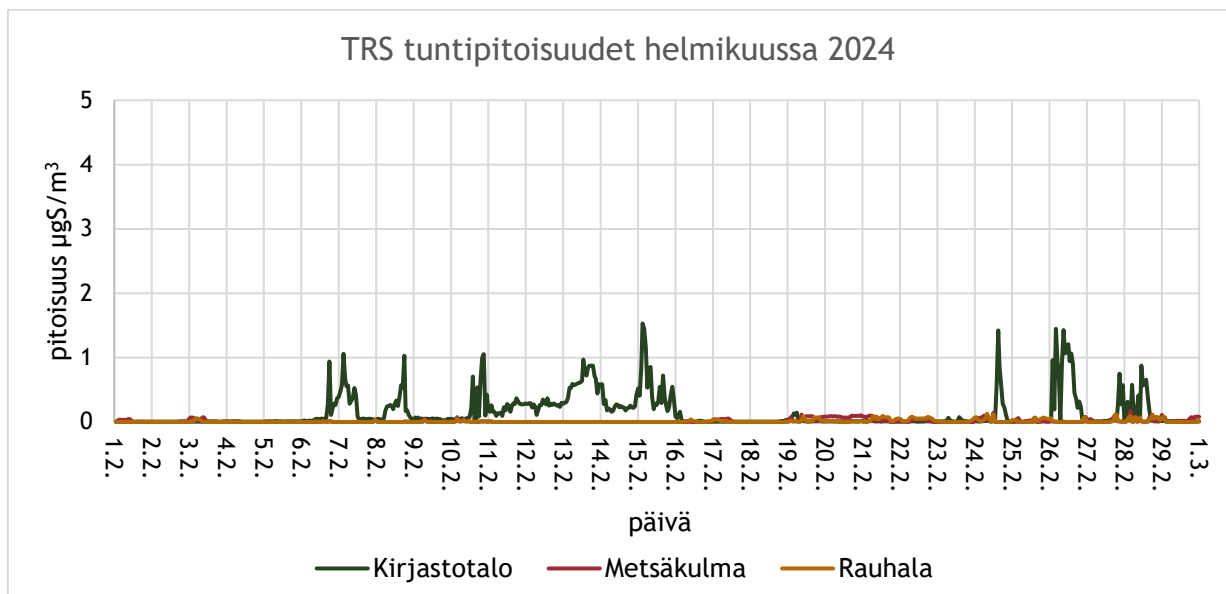
Kuva 4. TRS-tuntipitoisuudet ( \mu\text{gS}/\text{m}^3 ) helmikuussa 2024.
