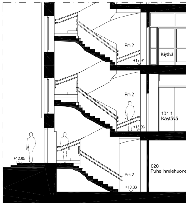
Leikkauspiirrosote B-B, porrashuone 2 - kellarin, 1. ja 2. kerros, 1:50
