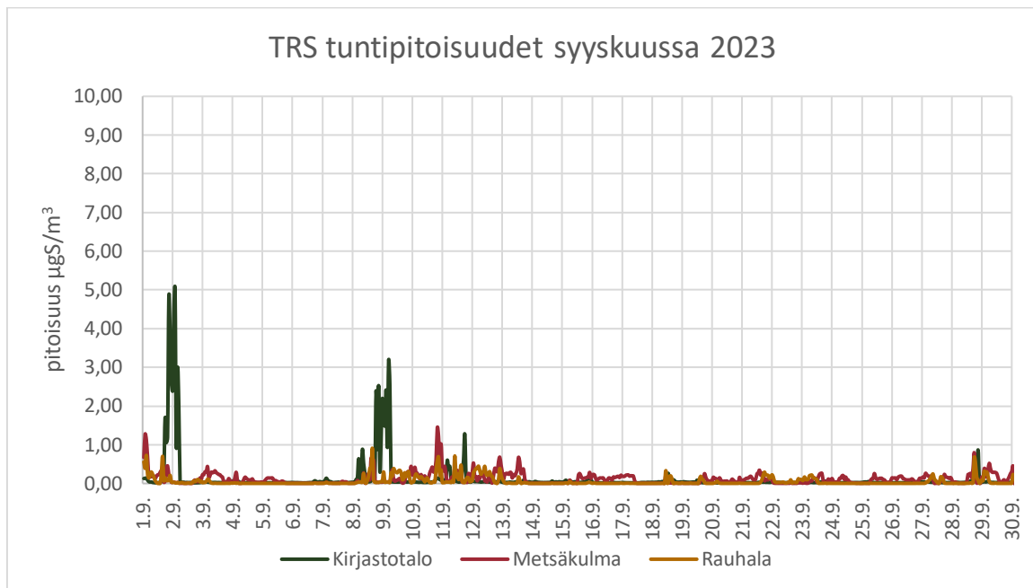
Kuva 5. TRS-tuntipitoisuudet ( \mu\text{gS}/\text{m}^3 ) 1.9. klo 01:00 -1.10. klo 00:00. Tuntipitoisuus \geq 3 \mu\text{gS}/\text{m}^3 on tunnistettava haju. Tuntipitoisuus \geq 1 \mu\text{gS}/\text{m}^3 on juuri aistittava eli hajukynnystaso .
