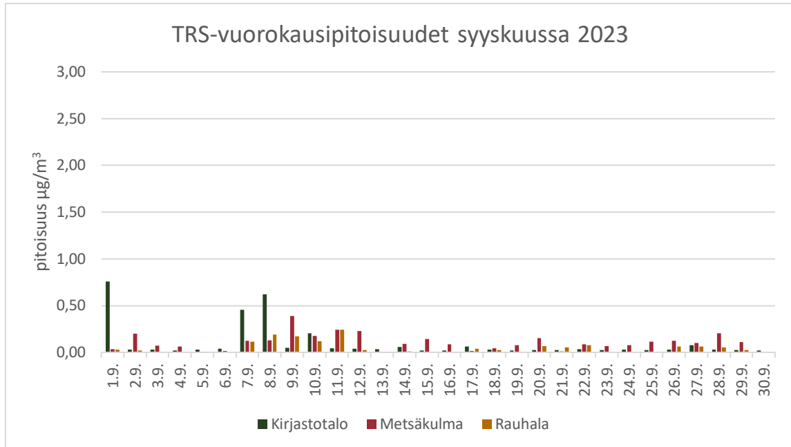
Kuva 4. TRS-vuorokausipitoisuudet ( \mu\text{gS}/\text{m}^3 ) syyskuussa 2023. Vuorokausiohjearvo on 10 \mu\text{gS}/\text{m}^3 (vertailuarvo kk:n 2. korkein).
