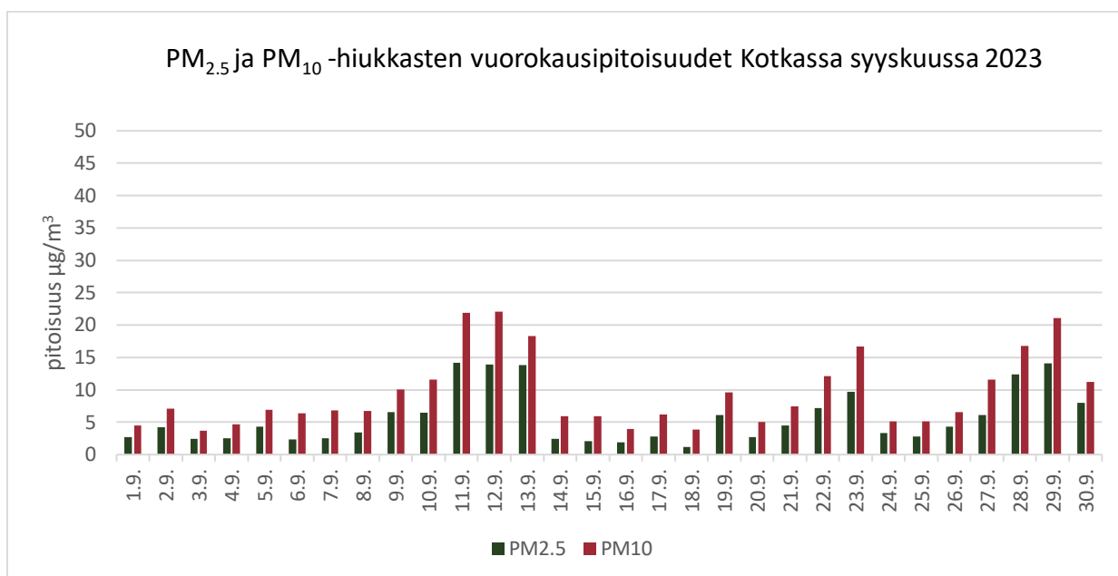
Kuva 3. Kirjastotalon PM 2.5 ja PM 10 -hiukkasten vuorokausipitoisuudet (µg/m 3 ) syyskuussa 2023. PM 10 vrk-ohjearvo on 70 µg/m 3 ja raja-arvon lukuarvo 50 µg/m 3 . WHO:n PM 10 vrk-ohjearvo on 45 µg/m 3 , PM 2.5 vuosiohjearvo on 5 µg/m 3 ja vrk-ohjearvo 15 µg/m 3 .
