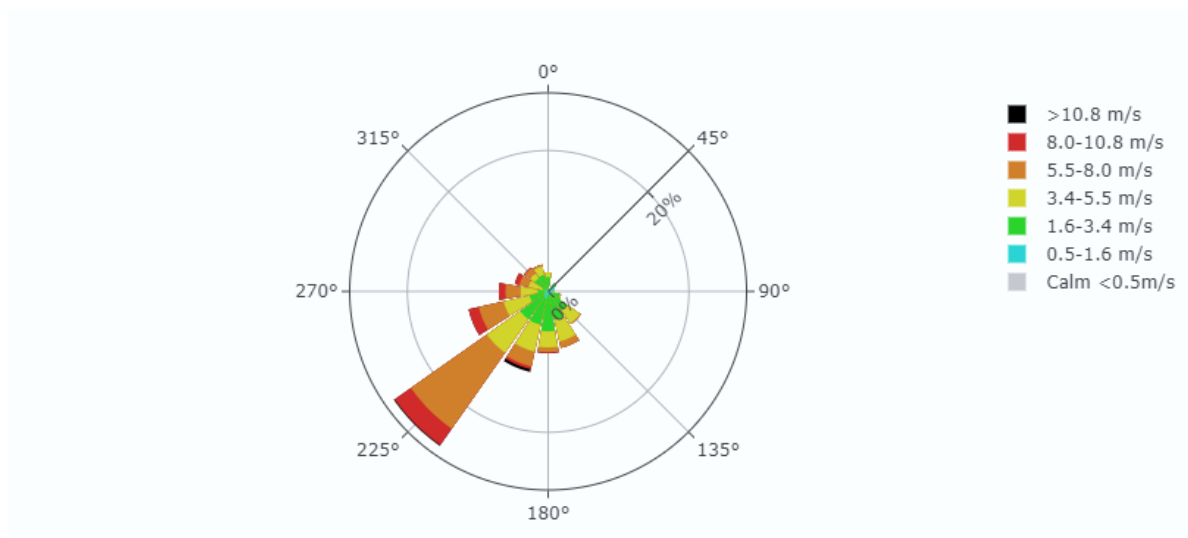
Kuva 1. Tuulen suunta- ja nopeusjakauma syyskuussa 2023. Tyyntä alle 0.5 m/s 0 % ajasta (Tuuliruusu = mistä tuulee).
